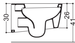
Vaso Sospeso Wall-hung Wc 36x54 cm
