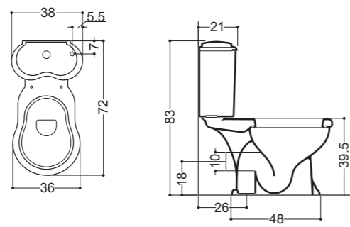
Vaso Monoblocco Suolo / Parete Monobloc Wc Floor / Wall 34x65 cm
