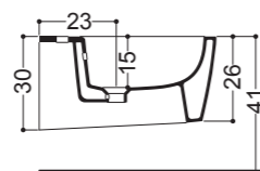
Bidet Sospeso Wall-hung Bidet 36x54 cm
