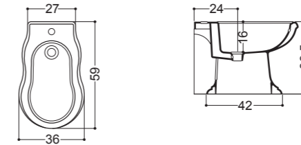
Bidet Terra Bidet 36x59 cm
