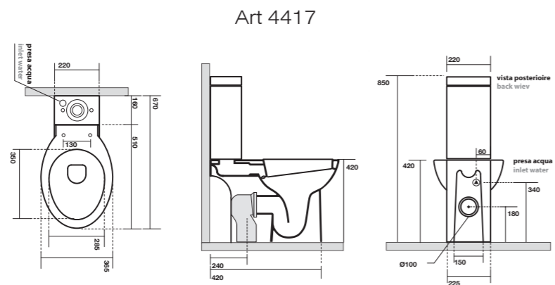
Vaso Monoblocco Monobloc Wc 36,5x67 cm
