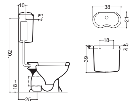
Art 06052 Cassetta Zaino Low level cistern 38x45,5 cm
