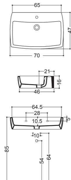
Lavabo Appoggio Overtop Basin 70x47 cm
