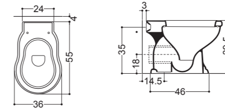
Vaso Terra Suolo / Parete Wc Floor / Wall 36x55 cm
