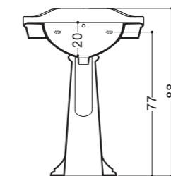
Lavabo angolare Corner Basin 60x48 cm
