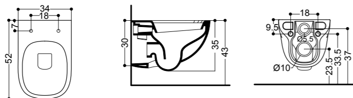
Vaso Sospeso Wall-hung Wc 34x52 cm
