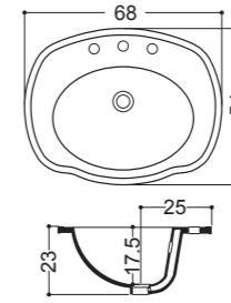
Lavabo incasso Inset Basin 68x54 cm
