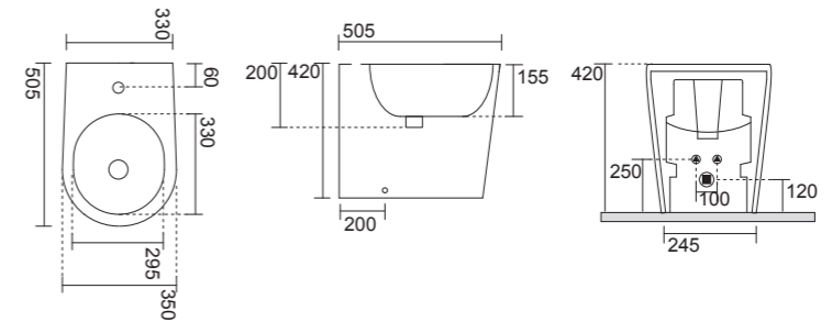
Bidet Terra BTW Bidet 33x50 cm
