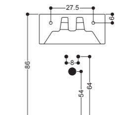
WSB55 Lavabo Sospeso monoforo con foro troppopieno Wall-hung Basin 1 hole with overflow 44x25 cm
