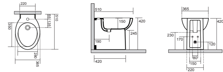
Bidet Terra BTW Bidet 36,5x51 cm
