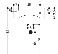
WSB57 Lavabo Sospeso monoforo con foro troppopieno Wall-hung Basin 1 hole with overflow 42x30 cm
