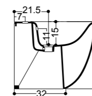
Bidet Terra BTW Bidet 34x52 cm
